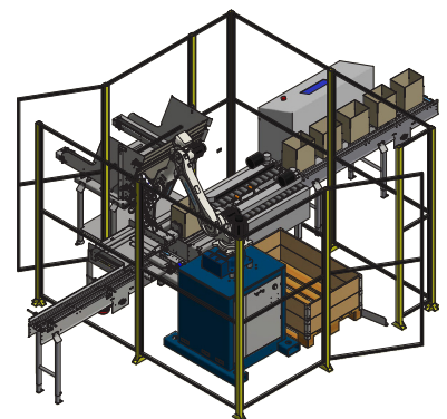
RobPack version 1, med dobbeltværktøj og standard sikkerhedshegn.
