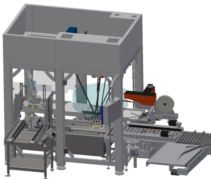
Rob modulerne kan samles - Her ses en RobPack celle, der rejser kasser, som fyldes af en RobFlex robot. Kassen lukkes og tapes automatisk efter opfyldning.
